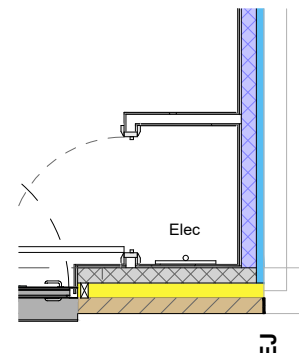
3 Mid Tce Elec Meter 1 : 50
